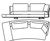
822-20-AS_L01_R04 B 274 T 123 H 85/87 SH 43/45 ST 60 AH 60/62
