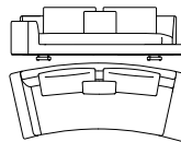
822-25-FS_L03_R01 B 319 T 127 H 85/87 SH 43/45 ST 60 AH 61/63
