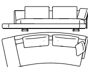
822-25-AS_L01_R04 B 304 T 124 H 85/87 SH 43/45 ST 60 AH 60/62
