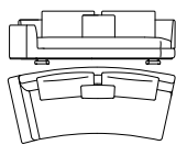
822-25-AS_L03_R00 B 268 T 121 H 85/87 SH 43/45 ST 60 AH 61/63
