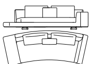
822-25-AS_L01_R03 B 319 T 127 H 85/87 SH 43/45 ST 60 AH 61/63
