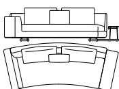
822-25-FS_L03_R07 B 302 T 123 H 85/87 SH 43/45 ST 60 AH 61/63
