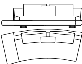
822-25-AS_L01_R00 B 299 T 124 H 85/87 SH 43/45 ST 60
