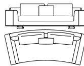
822-25-FS_L03_R03 B 288 T 124 H 85/87 SH 43/45 ST 60 AH 61/63
