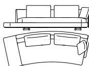
822-25-FS_L01_R04 B 304 T 124 H 85/87 SH 43/45 ST 60 AH 60/62
