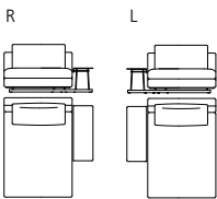
821-10 RE_L00_R07 B 158 T 177 H 85/87 SH 43/45
