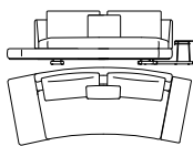
822-20-AS_L01_R07 B 303 T 123 H 85/87 SH 43/45 ST 60
