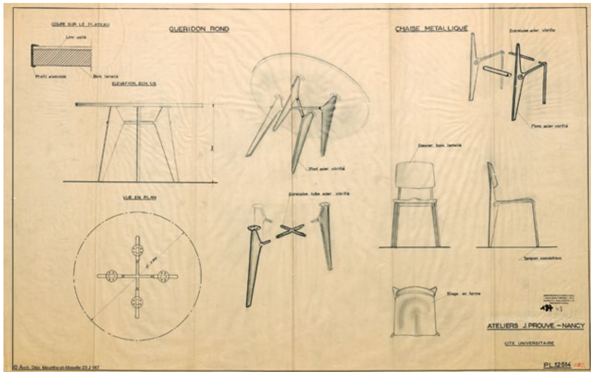
Technische Zeichnung des Tisches «Guéridon rond» und des «Chaise métallique», einer Version des Stuhls Standard, ca. 1950.
