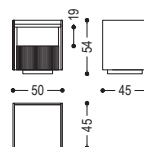
REVO NIGHT TABLE 2.1 CM: L. 50 · P. 45 · H. 54
