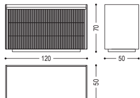
REVO NIGHT DRESSER 1 CM: L. 120 · P. 50 · H. 70
