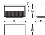
REVO NIGHT TABLE 2.2 CM: L. 90 · P. 45 · H. 54
