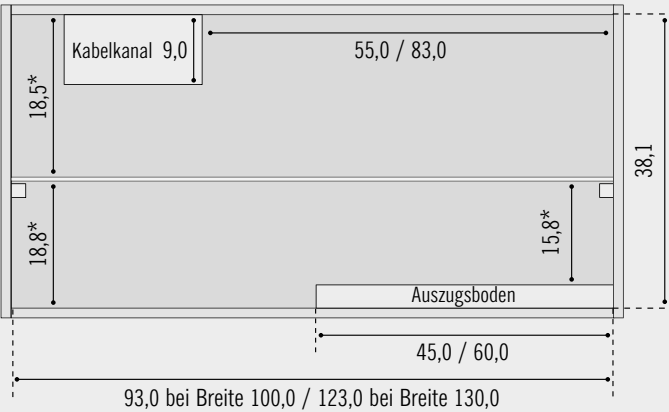
Innenmaße 2R – Sicht von vorn
