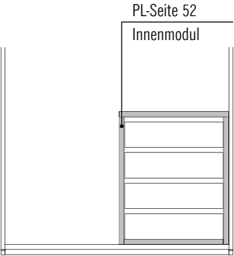
Das Innen-Modul besteht aus zwei Seiten, einem Oberboden und einem Unterboden sowie einer Rückwand. 4 oder 6 Innenschubkästen in 15 cm Höhe sind separat zu bestellen. Alternativ gibt es 7,5 und 30 cm hohe Innenschubkästen.
