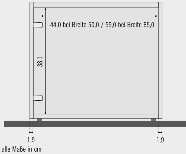
Innenmaße 2R – Sicht von vorn
