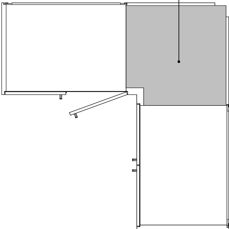
Seite 32 Eckelement mit Front-Eckleiste
