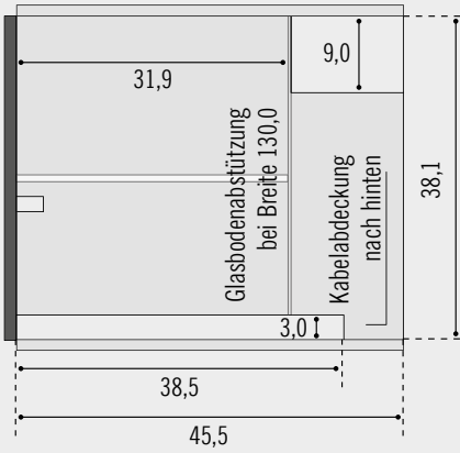
Innenmaße 2R – Sicht von der Seite
