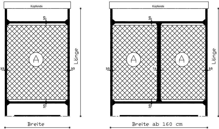
Schwebebett mit gewölbttem Kopfteil - Maße in cm, A = Innenmaß
