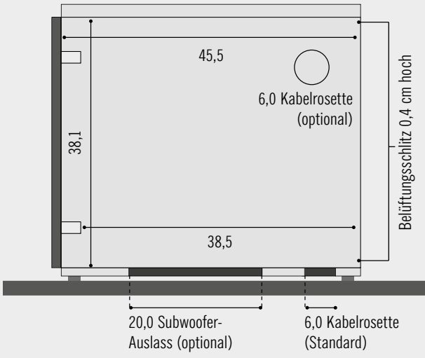
Innenmaße 2R – Sicht von der Seite
