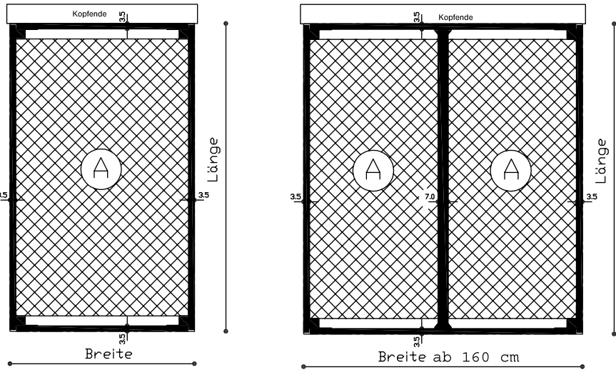
Bett mit Füßen oder Sockel mit gewölbttem Kopfteil - Maße in cm, A = Innenmaß
