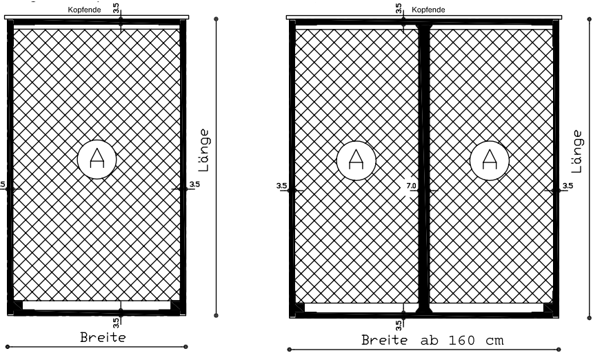
Bett mit Füßen oder Sockel mit geradem Kopfteil - Maße in cm, A = Innenmaß
