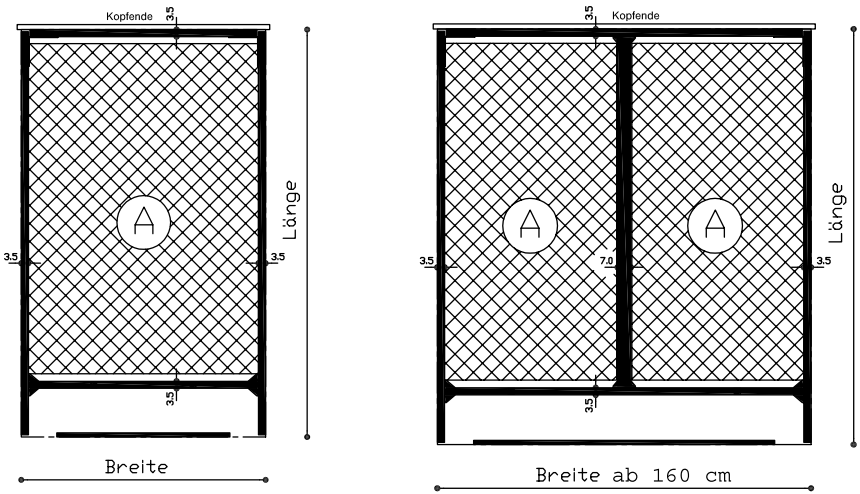
Bett schwebend mit geradem Kopfteil - Maße in cm, A = Innenmaß
