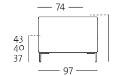
K-H-SOB 185 (Übertief) K-H-ASO 185 (Übertief)
