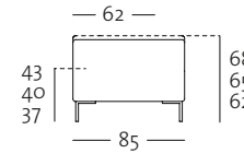
K-SOB 185 K-ASO 185
