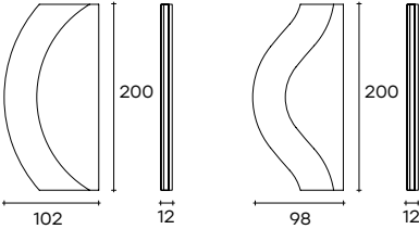
VERSIONE MODULARE / MODULAR VERSION
